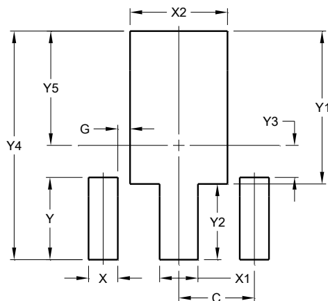
SOT89
