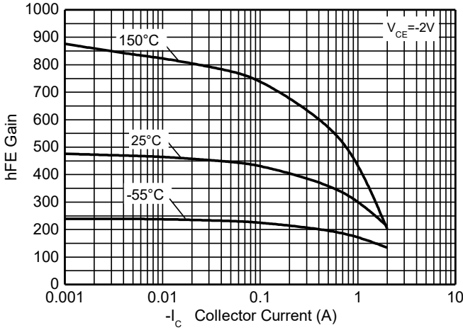
Fig. 5 hFE \ v \ I_C
