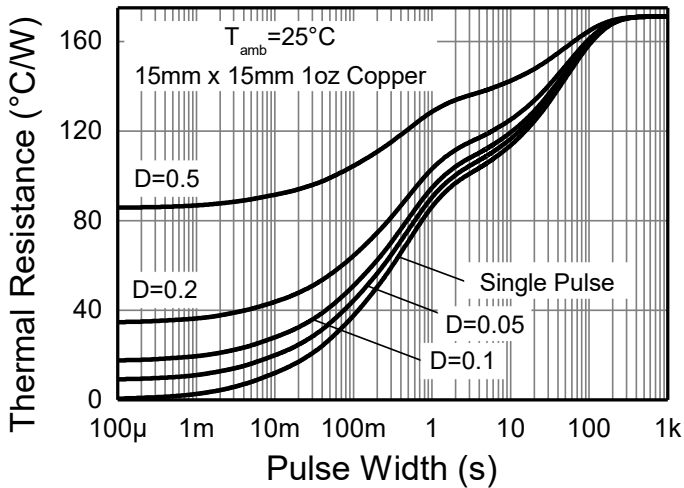
Fig. 3 Transient Thermal Impedance
