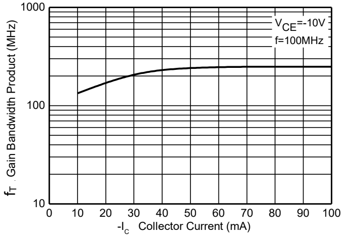
Fig. 11 f_T v I_C
