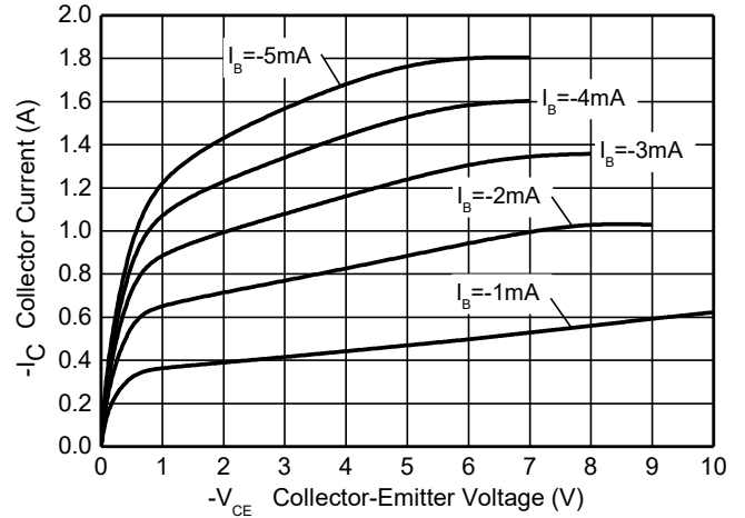
Fig. 6 I_C \ v \ V_{CE}
