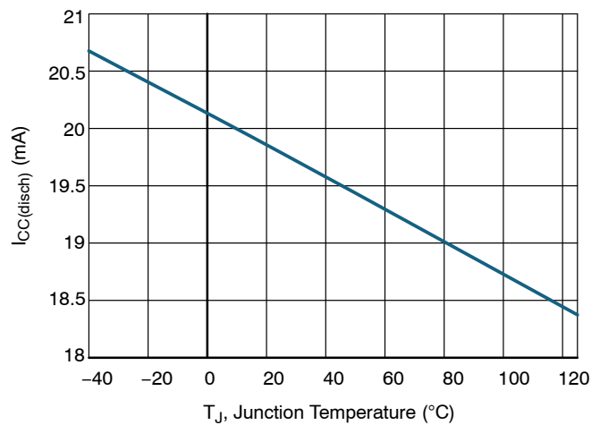
Figure 43. I CC(disch) vs. Temperature
