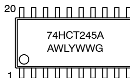
SOEIAJ-20
