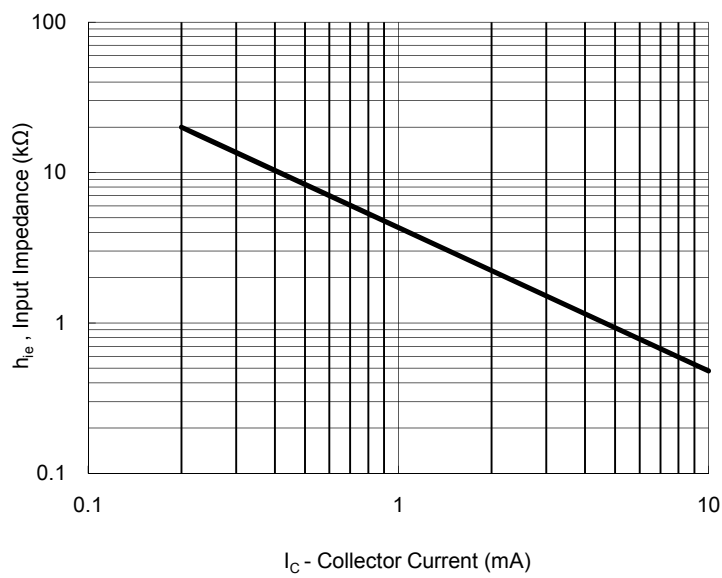
Fig. 9 Input Impedance
