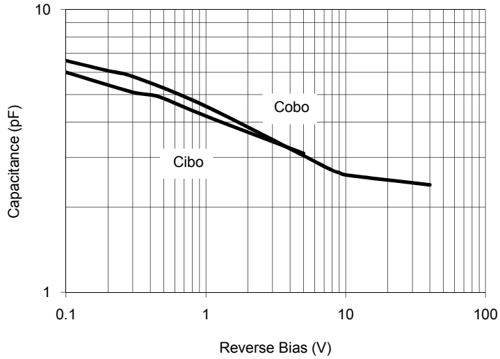
Fig. 1 Capacitance
