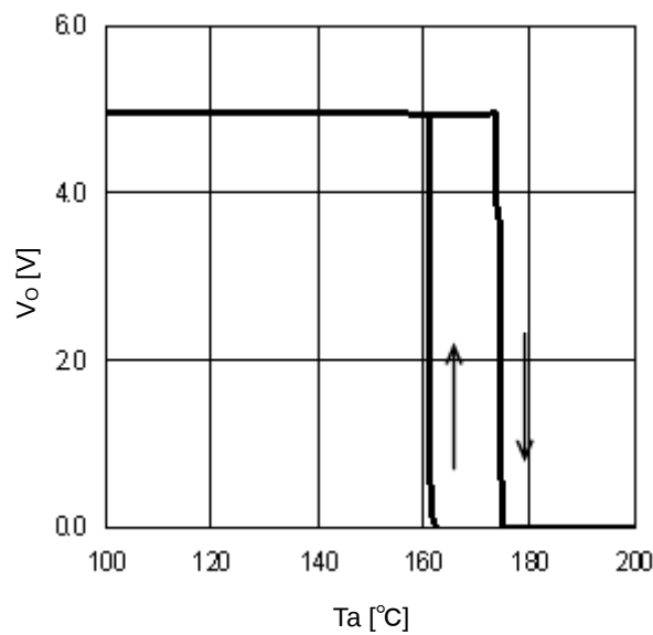
Figure 28. TSD ( I_o=0\text{mA} )
