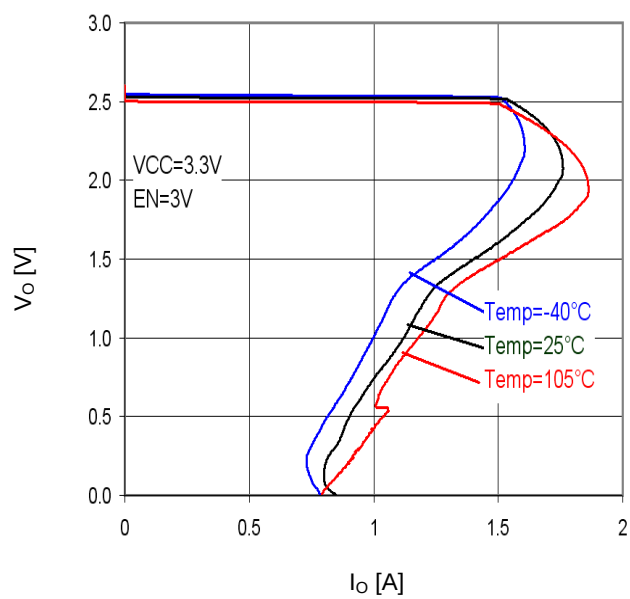
Figure 29. I_o - V_o
