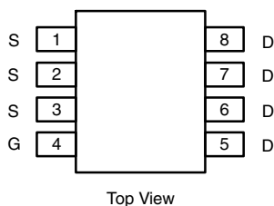
SO-8
