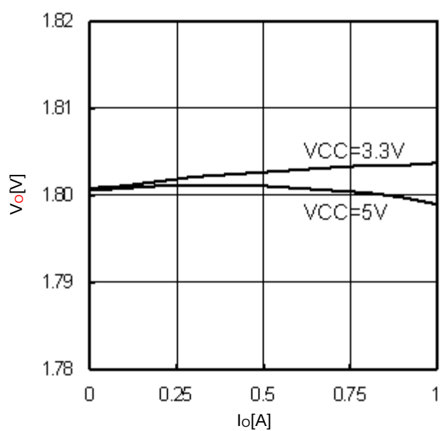
Fig.17 Io-Vo (Vo=1.8V)
