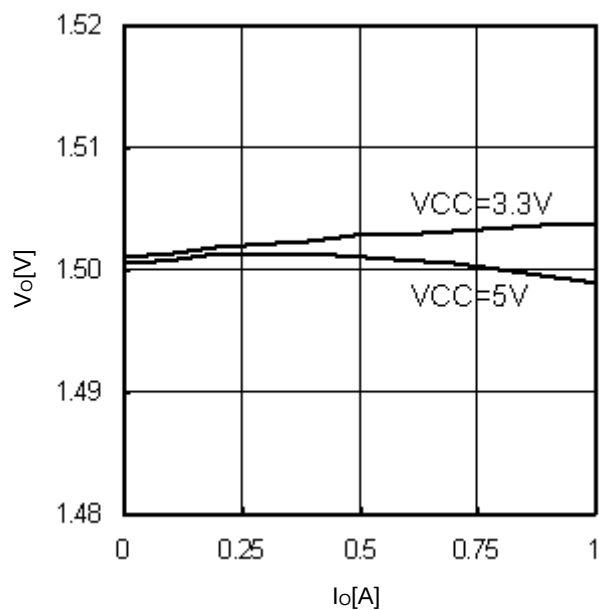
Fig.16 Io-Vo (Vo=1.5V)
