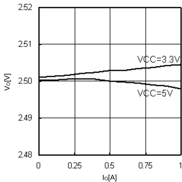
Fig.18 Io-Vo (Vo=2.5V)
