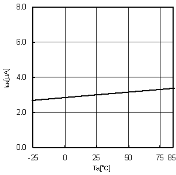
Fig.14 Ta-Ien
