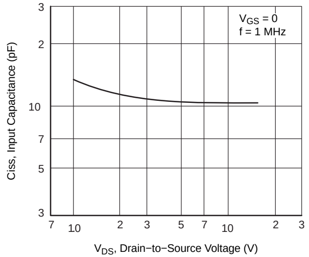
Figure 8. C_{iss} – V_{DS}
