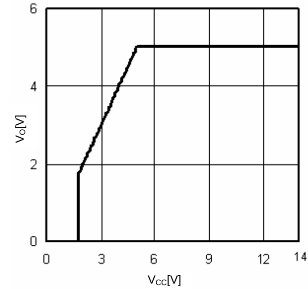
Fig.15 V_{CC}-V_O ( I_O=0\text{mA} )
