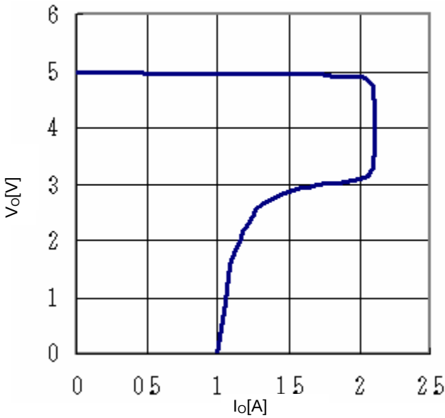
Fig.17 OCP
