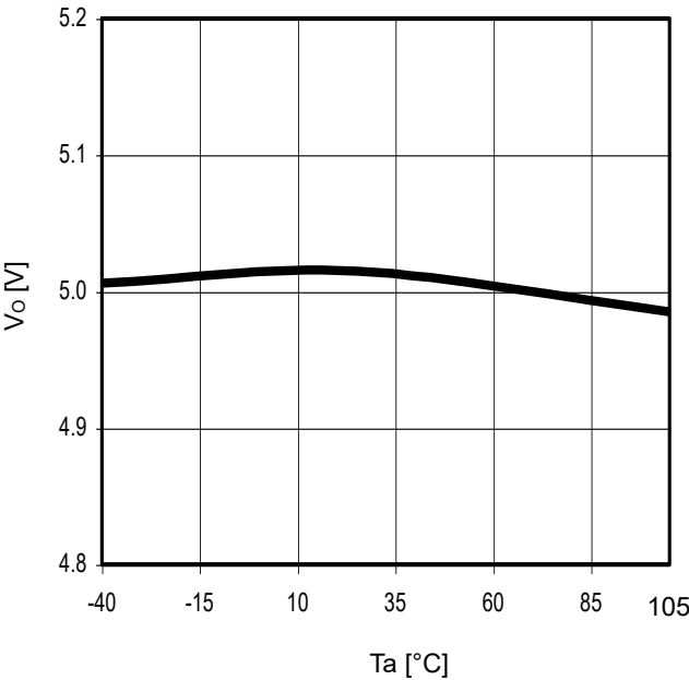
Fig. 21 Ta-V_O ( I_O=0mA )
