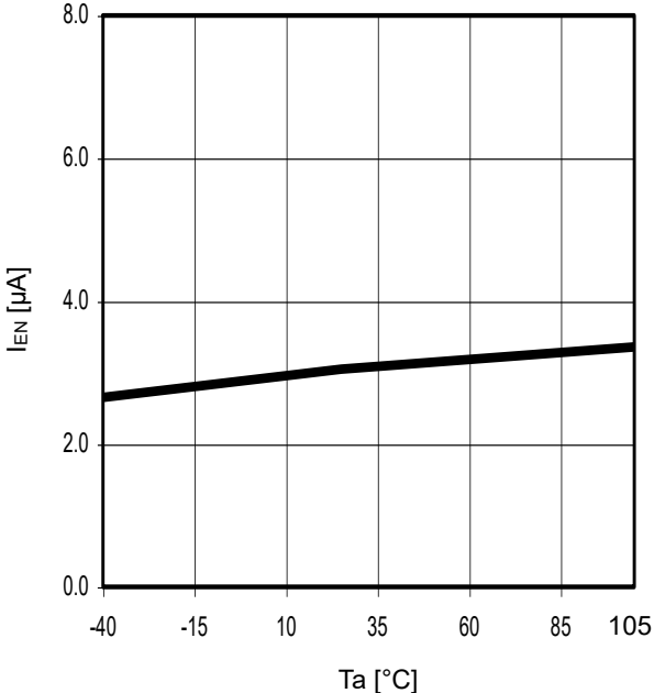
Fig. 24 T_a - I_{EN}
