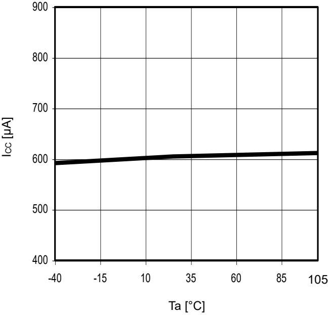
Fig. 22 Ta-I_{cc}
