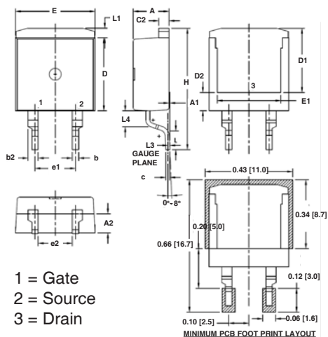
TO-263HV Outline
