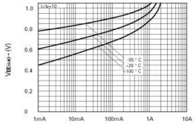
I_C -Collector Current V_{BE(sat)} v I_C
