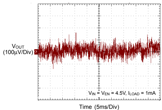
VOUT1 Noise
