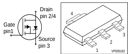
PG-SOT223
