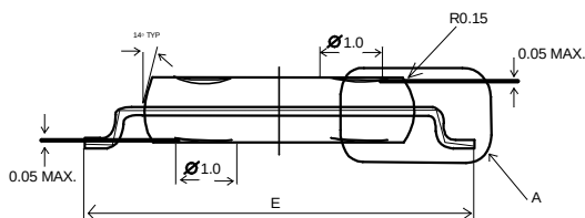
SECTION V-V
