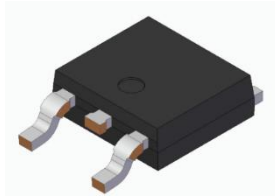
TO252 (DPAK)
