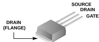
JEDEC TO-262AA
