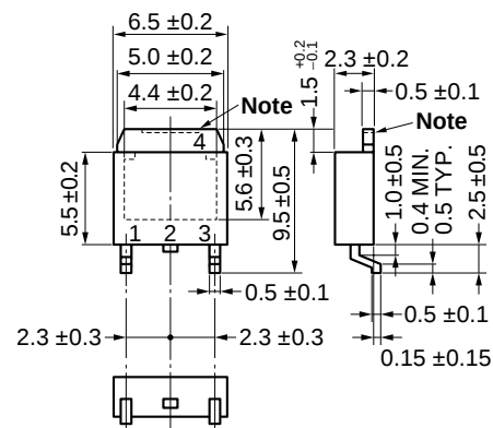
TO-252 (MP-3Z)
