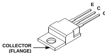
JEDEC TO-220AB
