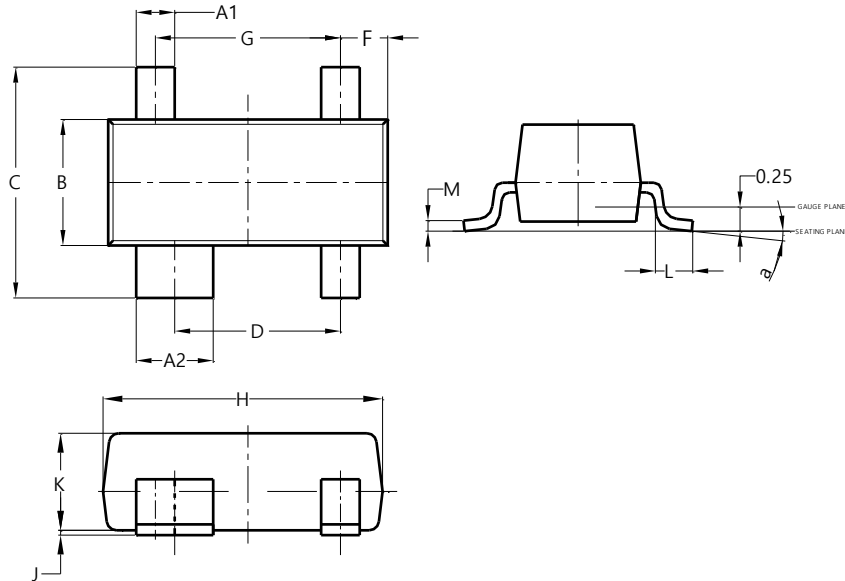
SOT143
