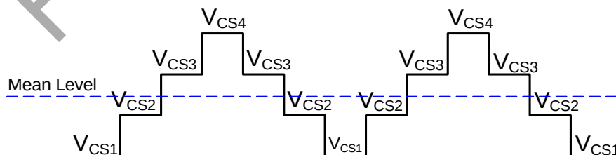
Figure 4. V_{CS} Jitter
