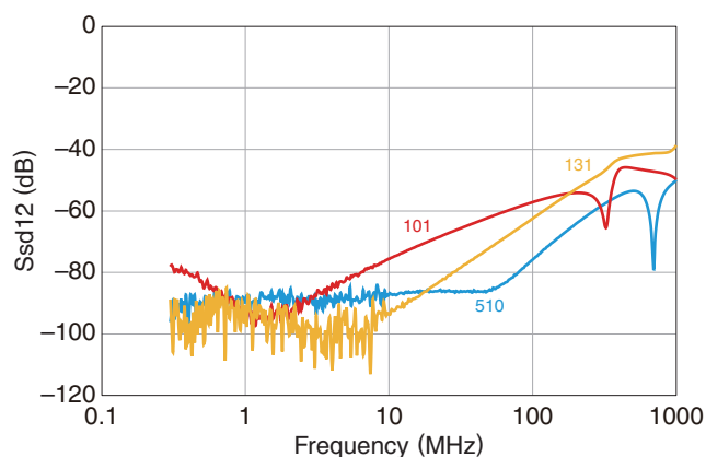
■ Ssd12
