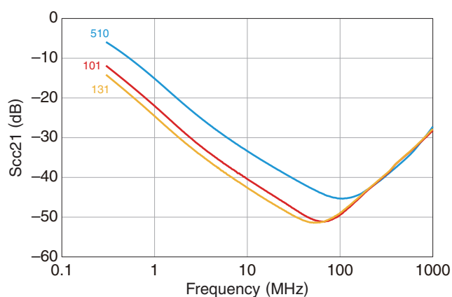
■ Scc21
