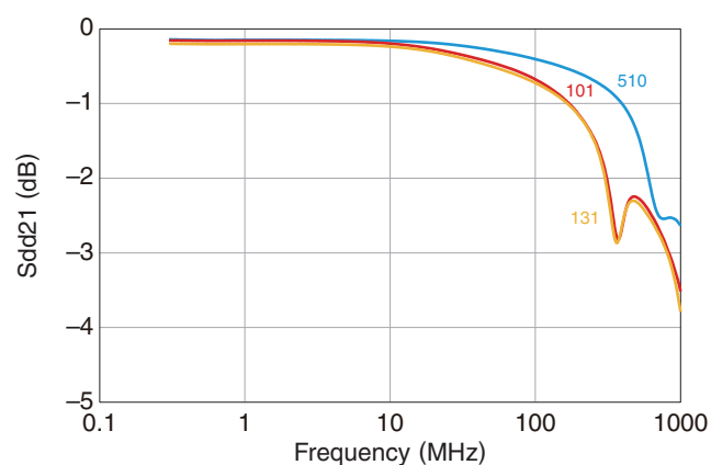
■ Sdd21
