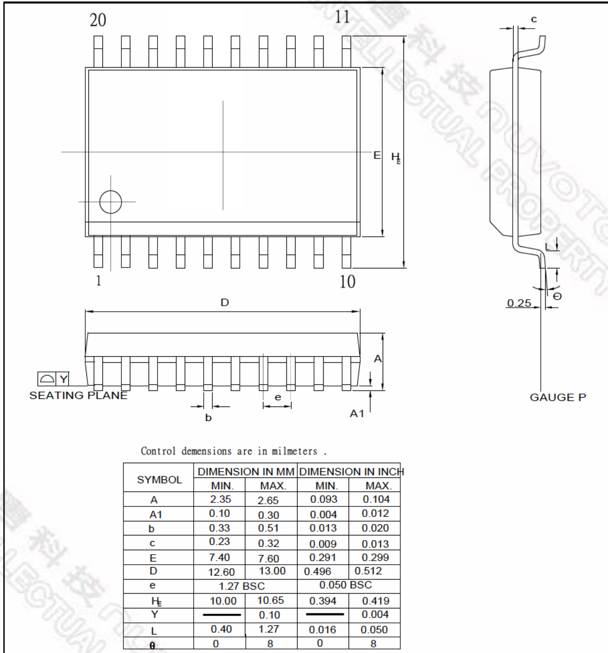
Figure 27-1: 20L SOP-300mil
