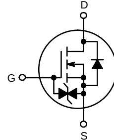
POWER MOSFET
