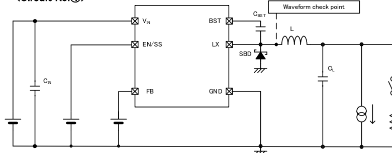
&lt;Circuit No.④&gt;
