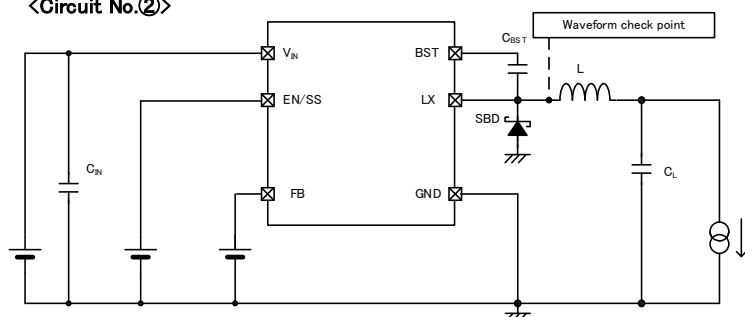
&lt;Circuit No.②&gt;
