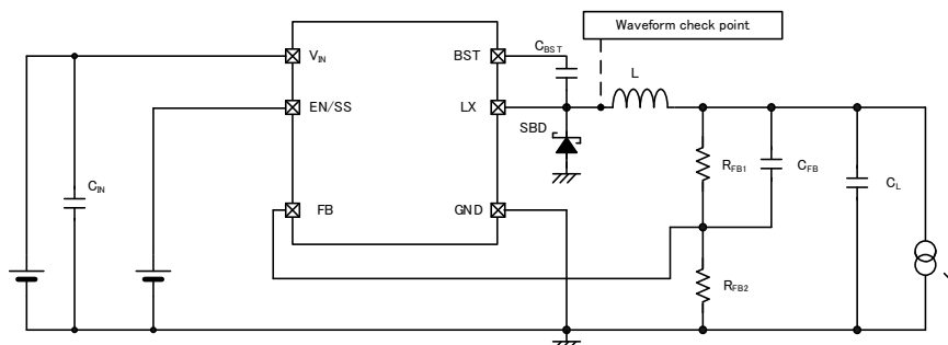
&lt;Circuit No.①&gt;
