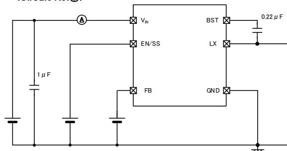
&lt;Circuit No.③&gt;
